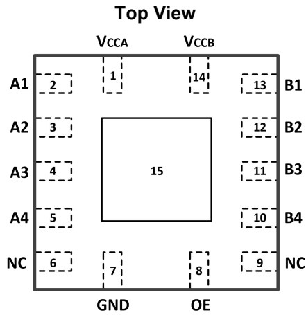
Fig.5-1. GT0104: QD (QFN3.5x3.5-14L) Package
